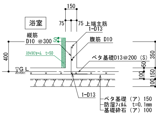
浴室内部基礎断面 S=1/30
