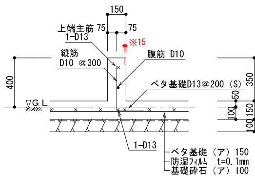
内部基礎断面 S=1/30
