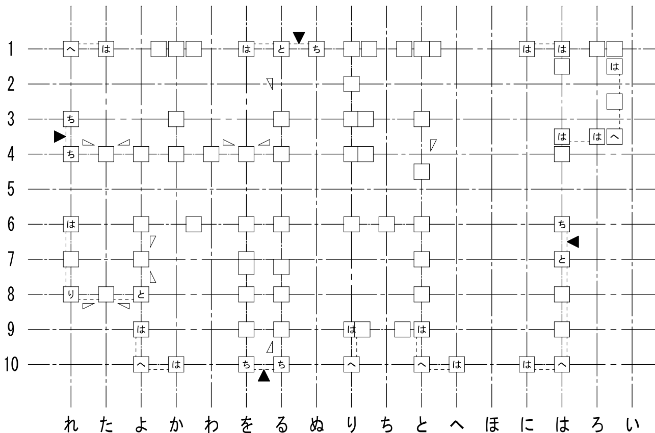
1 階柱壁伏図
