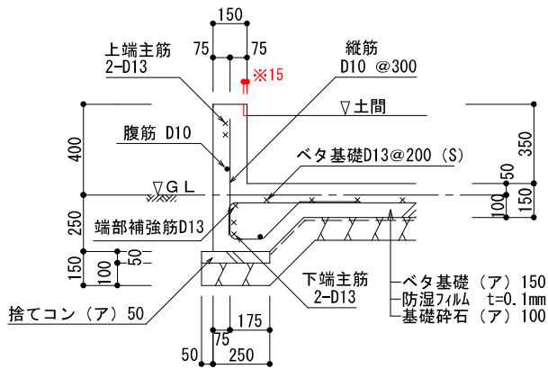
外周基礎断面 S=1/30
