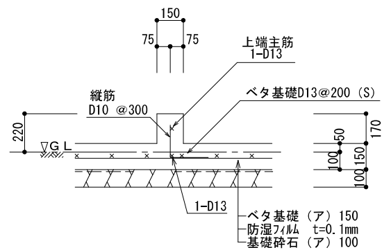
ポーチ下 内部部基礎断面 S=1/30
