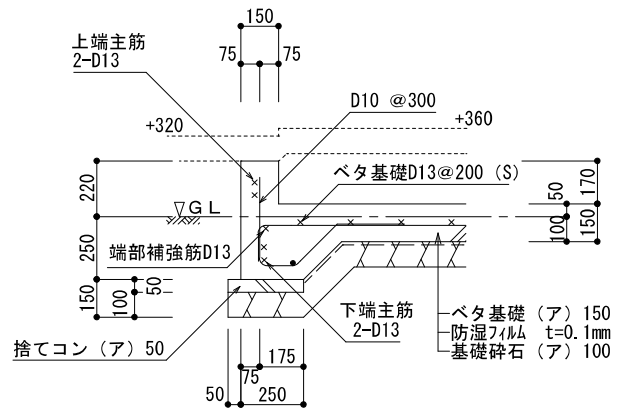
ポーチ下 外周部基礎断面 S=1/30
